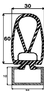
Coupe CM 2000
