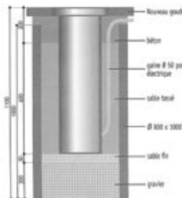
Exemple de schéma de fondation
