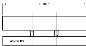
Verrou 70180 pour porte à 1 vantail
