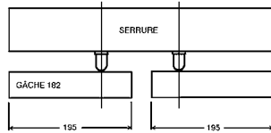
Verrou 70182 pour porte à 2 vantaux
